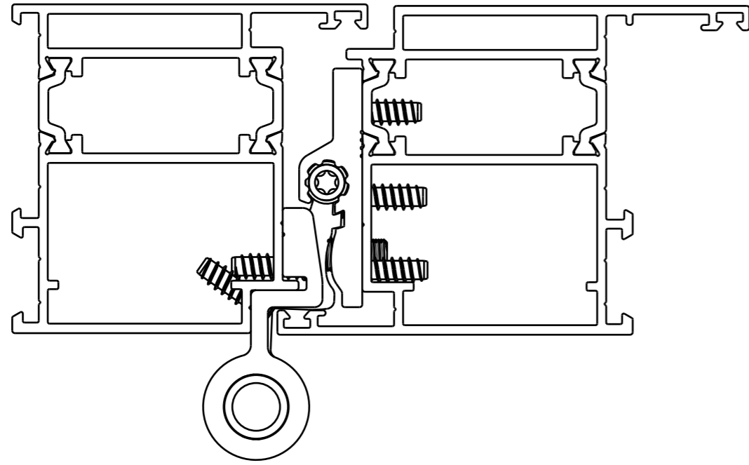
Nach innen öffnende Tür 62
