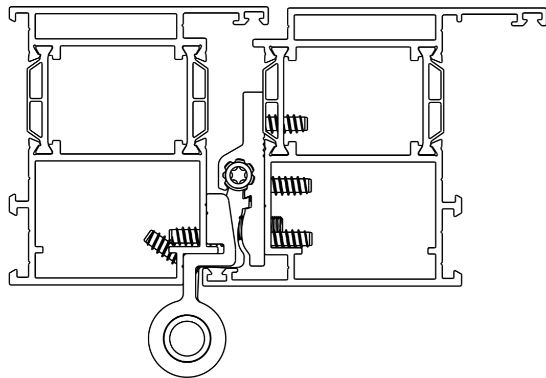
Nach innen öffnende Tür 72
