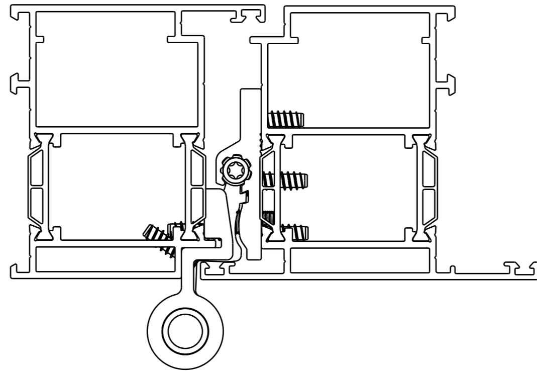
Nach außen öffnende Tür 72
