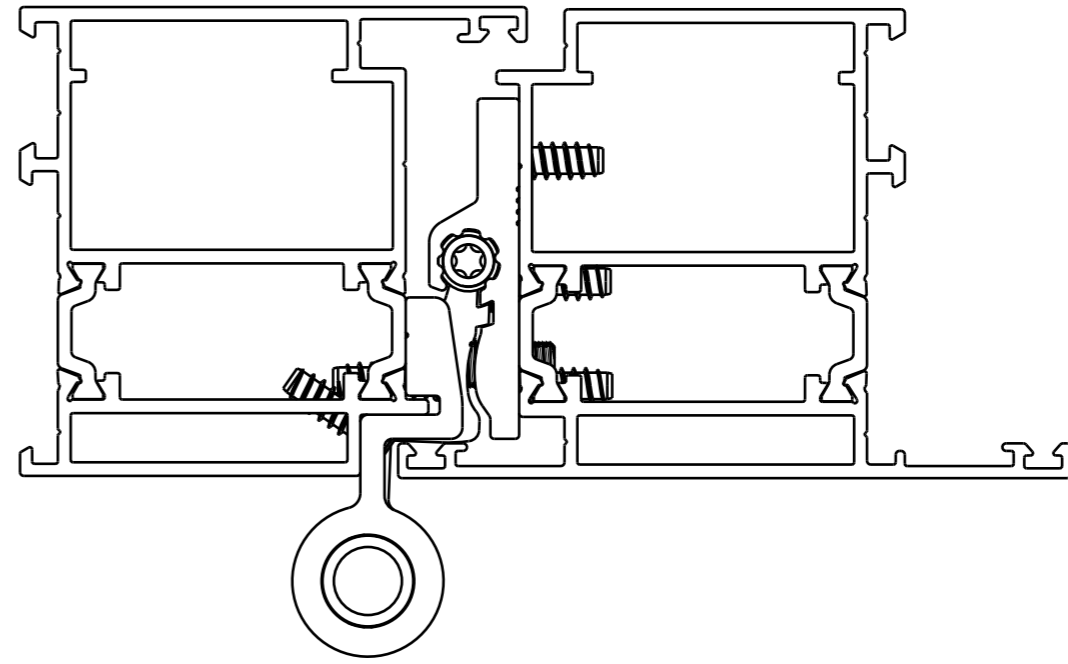
Nach außen öffnende Tür 62
