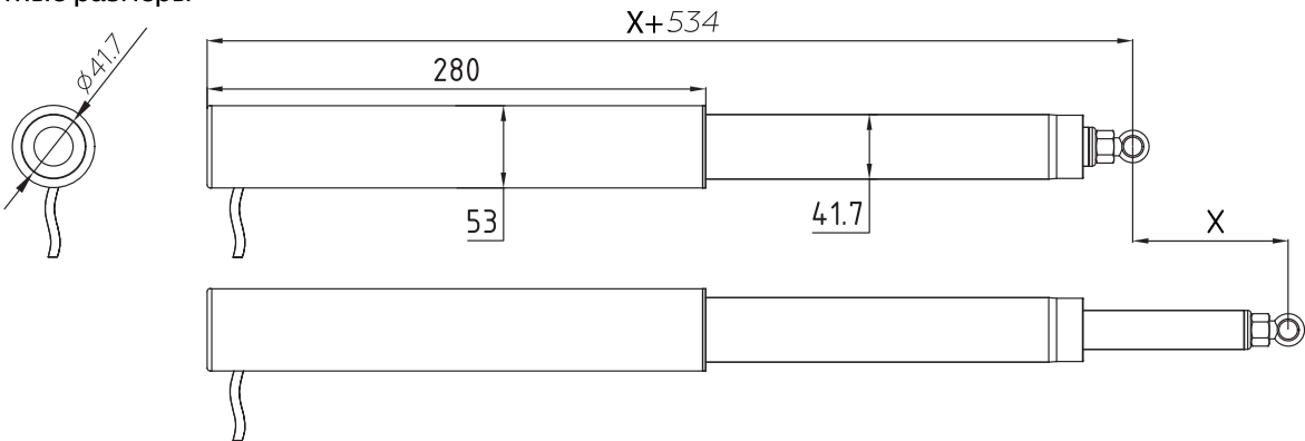
Примеры монтажа
