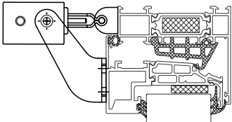
Открытие вовнутрь монтаж на створку
