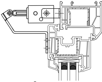
Открытие вовнутрь монтаж на раму
